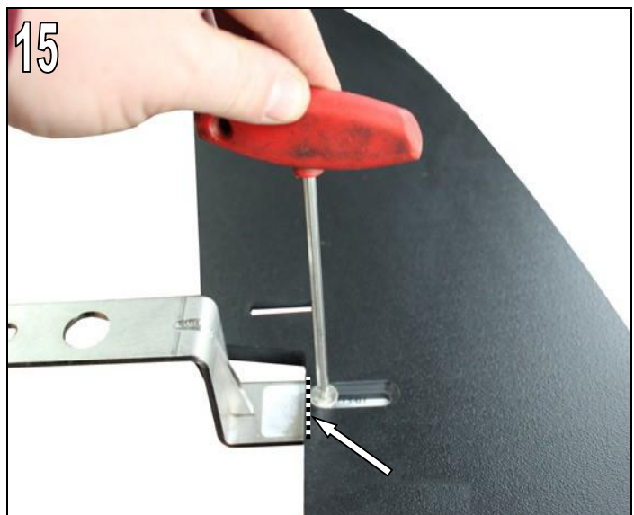
Abb. 15 AC Schnitzer Befestigungshalter mit der mitgelieferten Senkkopfschraube M6x10mm am AC Schnitzer Frontsplitter montieren und festziehen.
